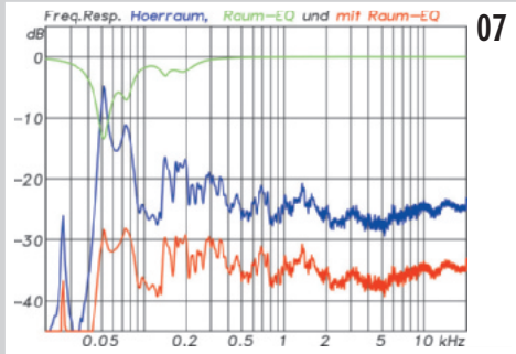
07 Gemittelte Frequenzgangmessung über je 30 Positionen für den linken und rechten Lautsprecher um den Hörplatz (blau). Unterhalb von 150 Hz sind die Raummoden gut zu erkennen. Aus den Messungen wurde ein EQ (grün) zur Raumkorrektur abgeleitet. Unten die gemittelte Kurve mit EQ (rot).
