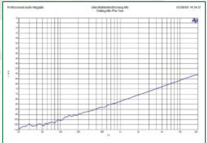
Die Gleichtaktunterdrückung erreicht ihr Maximum von -55 Dezibel bei 20 Kilohertz, was bei sehr langen Kabeln kritisch werden kann.
