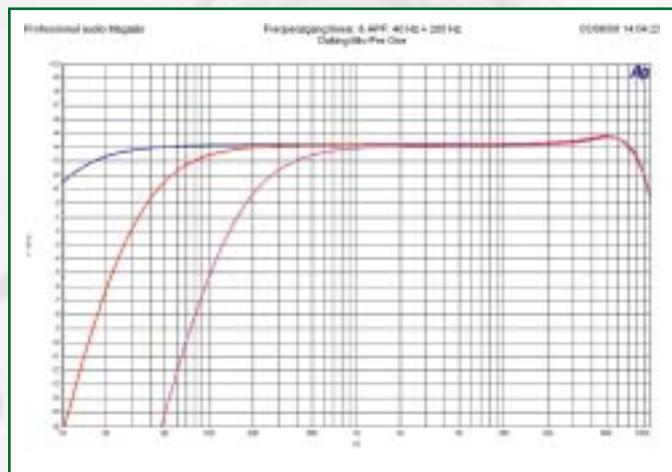
Der Übertragungsbereich ist innerhalb des Hörbereichs sehr linear. Ein leichtes Überschwingen bei 50 Kilohertz leitet den Pegelabfall ein, der bei 100 Kilohertz etwa drei Dezibel beträgt.
