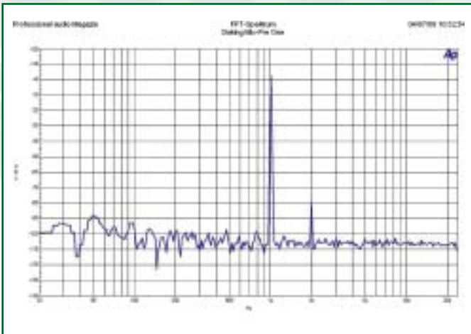
Das FFT-Spektrum ist mit unter -100 Dezibel sehr sauber. Leichte Unsauberkeiten liegen unter -80 Dezibel und fallen nicht weiter ins Gewicht.
