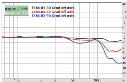
Sehr geringe Off-Axis-Verfärbungen für ein Großmembranmikrofon (Pegel angeglichen, die 0-dB-Linie repräsentiert die On-Axis-Response)
