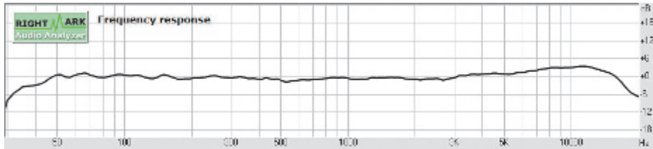
Die Messung unter praxisnahen Bedingungen zeigt einen sehr ausgeglichenen Frequenzgang.
